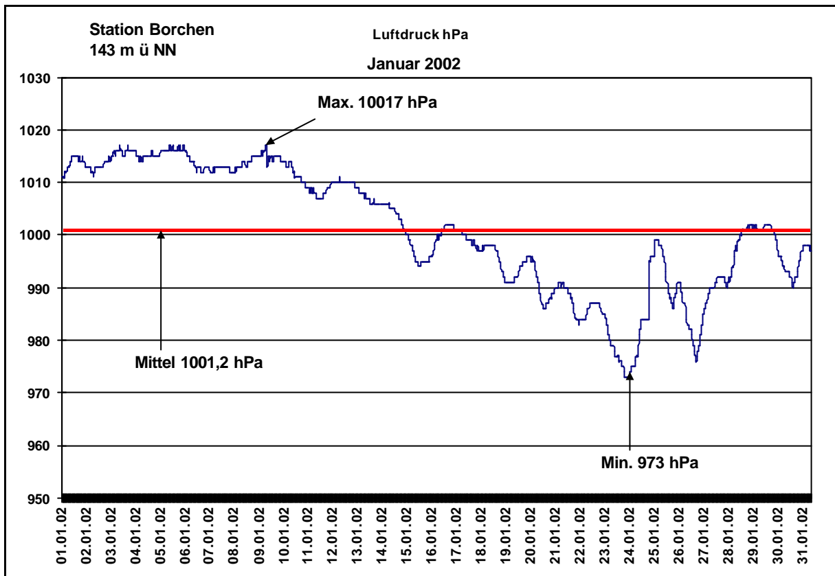
Abbildung Luftdruck: die Werte liegen um 20 hPa zu niedrig wegen fehlender Kalibrierung der Höhe
